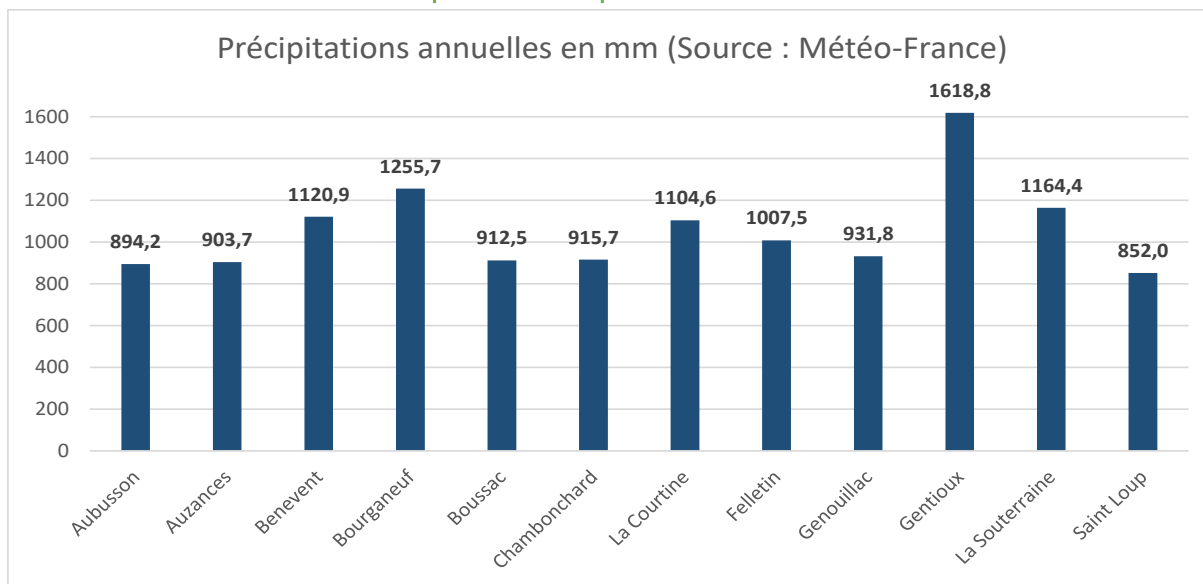
Figure 3 : Précipitations annuelles en mm (Source : Météo-France)
