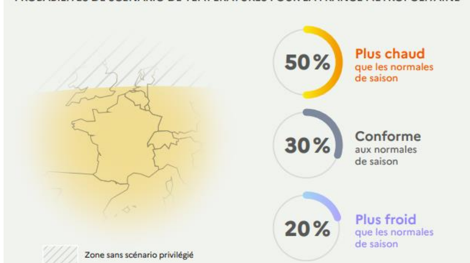
Figure 1 : Tendances à trois mois pour les températures (Source : Météo-France)
